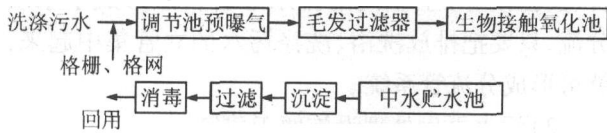
图 2 污水再生处理工艺
