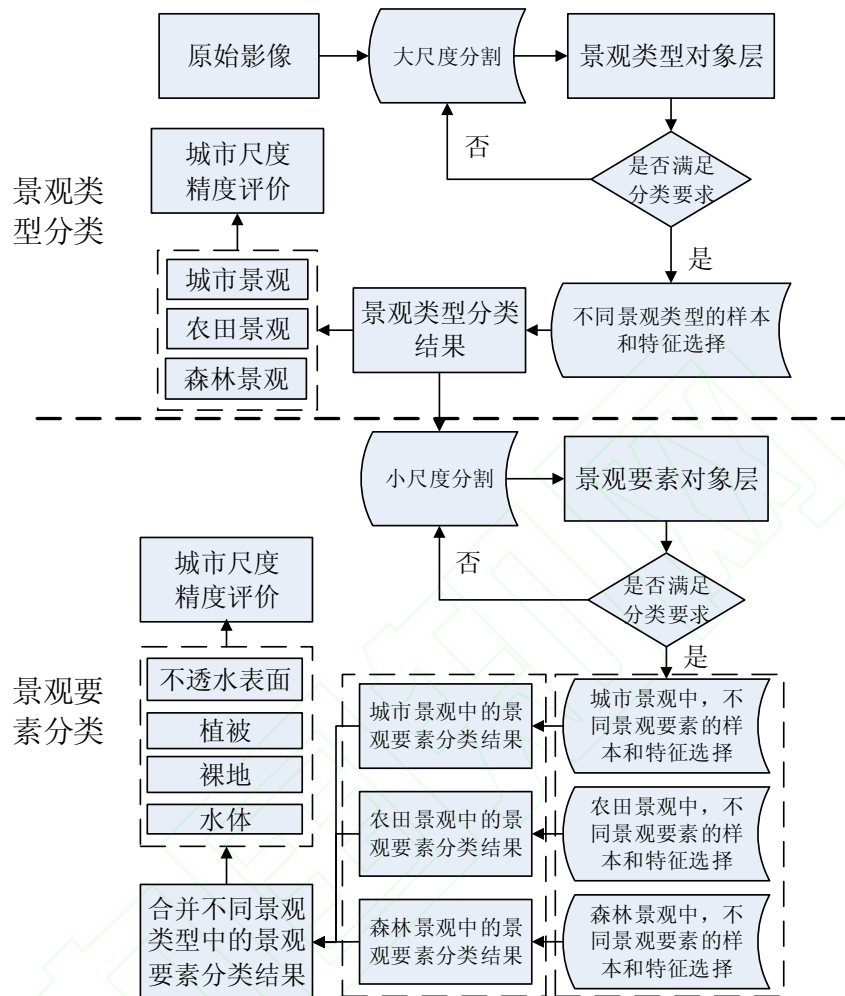
图 2 自上而下的分类流程
